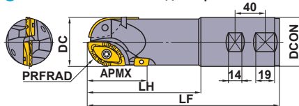
● Тип с хвостовиком Велдона (рис. 1)
