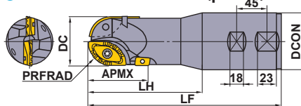
● Тип с хвостовиком Велдона (рис. 3)
