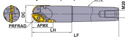
● Тип с конусом Морзе (рис. 6) МТ5
