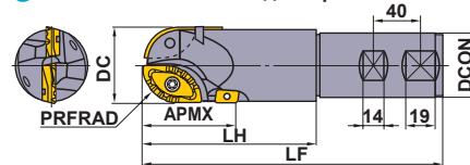
● Тип с хвостовиком Велдона (рис. 2)
