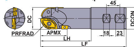
● Тип с хвостовиком Велдона (рис. 4)
